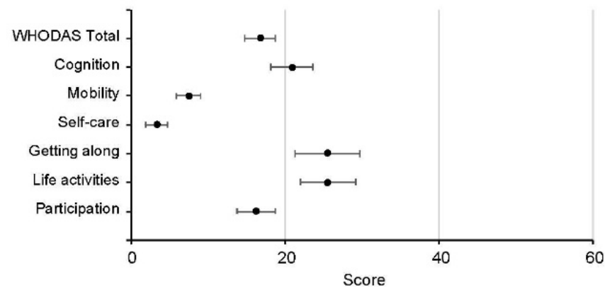
(D) SR LOCF=No, Achieved goal=No
