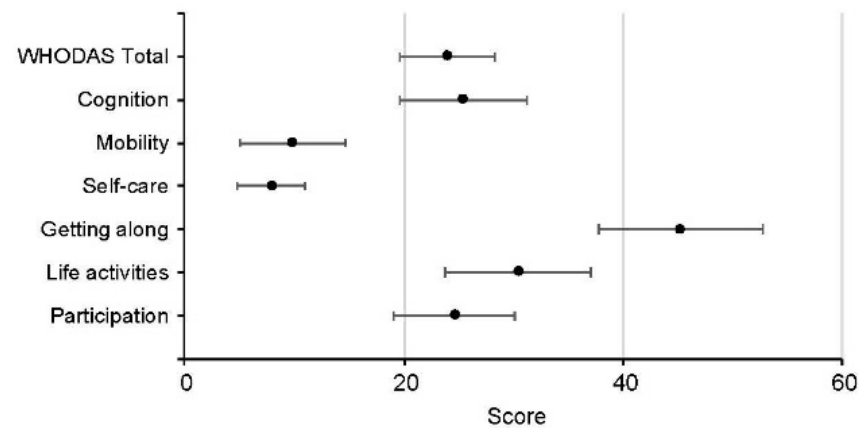
(D) SR LOCF=No, Achieved goal=No
